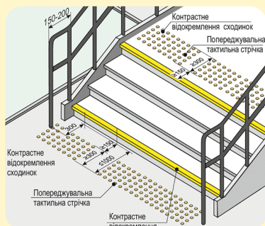
Приклад облаштування сходів (розміри вказані у мм)
