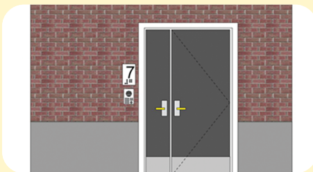
Приклад облаштування вхідних дверей (розміри вказані у мм)
