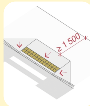
Приклад влаштування бордюрного пандусу (розміри вказані у мм)
