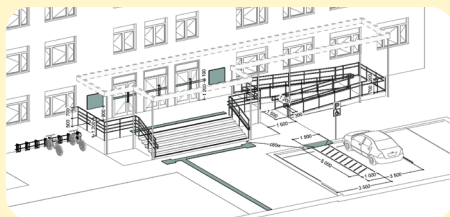
Схема облаштування шляху руху до входу у будівлю (розміри вказані у мм)
