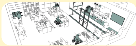
Приклад облаштування приміщення бібліотеки (розміри вказані у мм)
